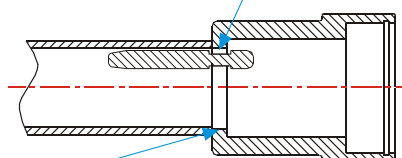
УПОРНАЯ ВТУЛКА, ОСНАЩЕННАЯ РОЛИКАМИ С ЖЕЛОБОМ
